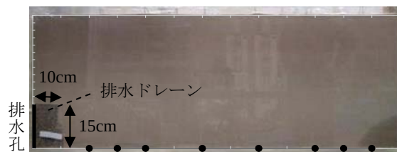
図 1 基礎地盤のみの実験の初期状態 (Case_1)
