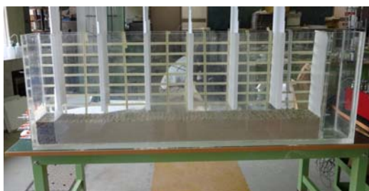
図 5 模型地盤の作成方法
