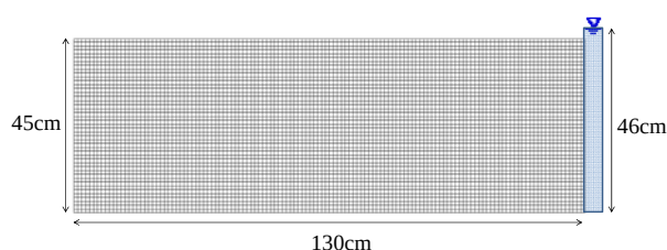
図 3 Case_1の解析断面
