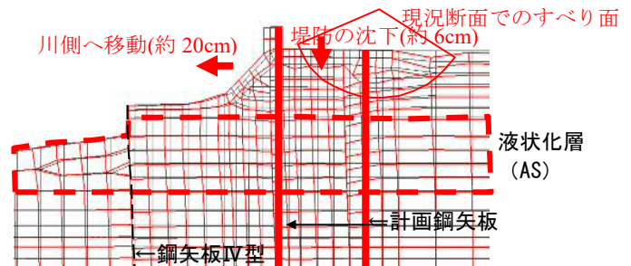
図-13 対策工断面変形図
