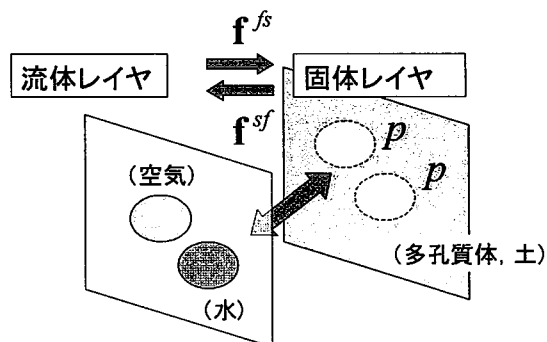
図-3 固体相（土）と流体相（液体、気体）との重ね合わせと相互作用
