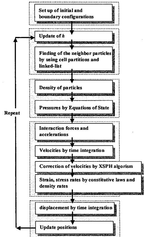
図-5 SPH 法による計算フロー
