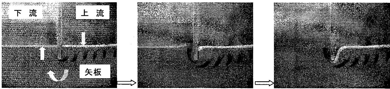
図-10 矢板周りの浸透破壊の実験の様子 (DO が飽和量を超えていない状態 (未飽和状態) の水) : 限界水位差 18cm を負荷した場合
